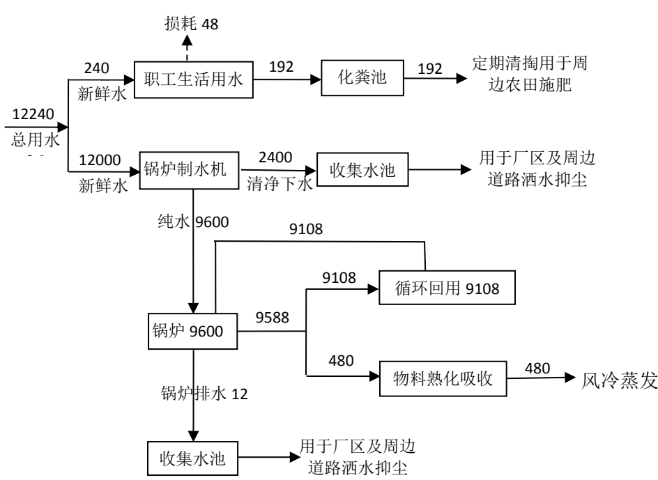
图 4 本项目水平衡图 单位：t/a
